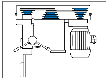
PU: Stufenscheiben V22 -V25
