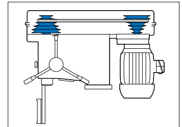
PU (E): Stufenscheiben mit elektronischem Geschwindigkeitsregler V22E-V25E
